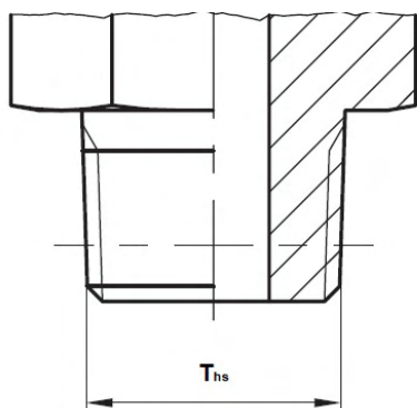
Filetto conico
